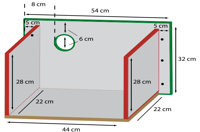
Fig. 5: Nido fissato orizzontalmente. Il tetto e la parete dietro sono piazzati sui bordi rossi. La superficie verde è piazzata contro il muro interno della costruzione.
